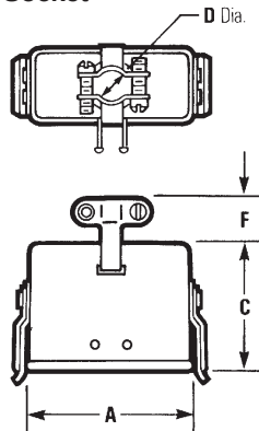
Socket
