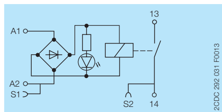
RB(R)111-24VUC
