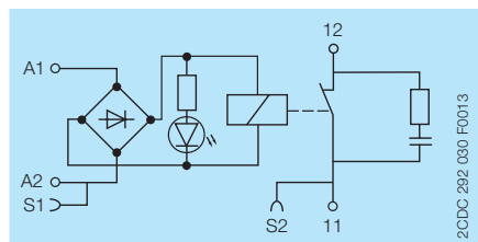
RB(R)101R - 24VUC
