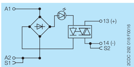
OB(R)OA
