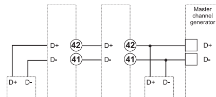
Fig. 29 Dupline port
