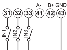
Fig. 27 Digital inputs
