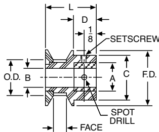
DOUBLE FLANGE 10-16 GROOVES
