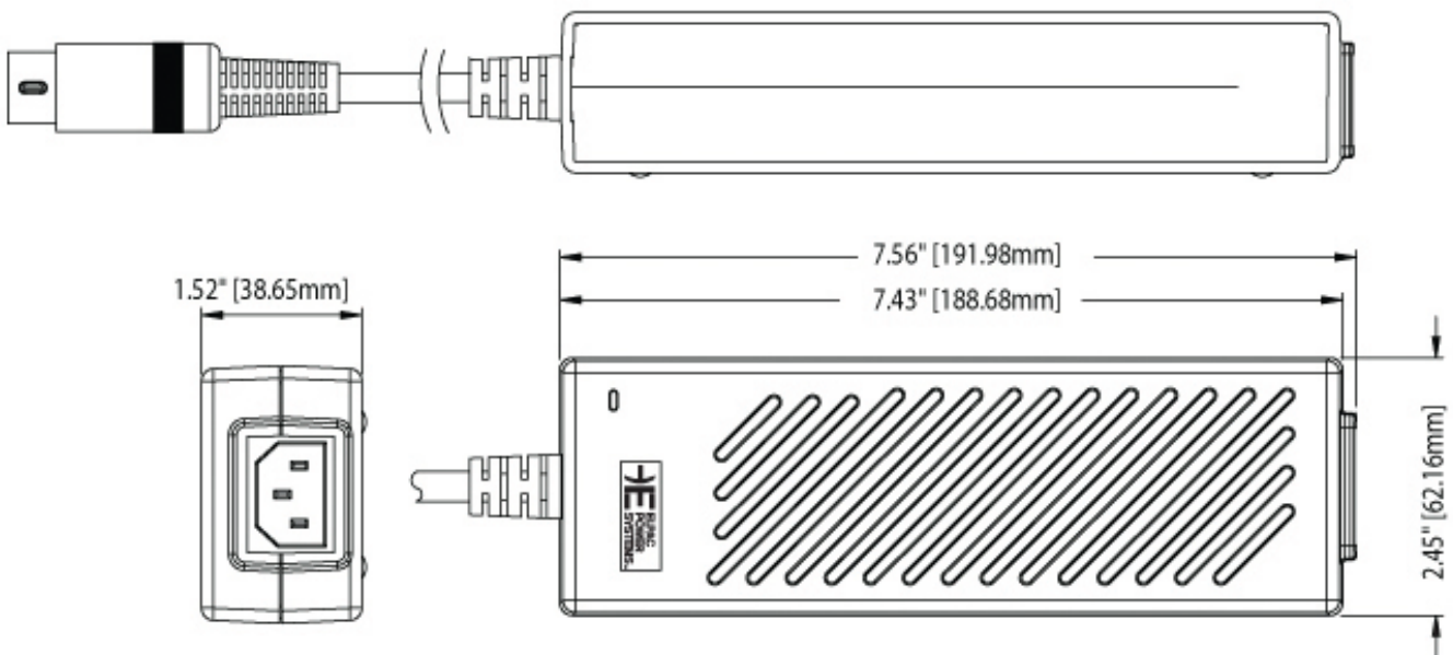
MWA120-DWG
