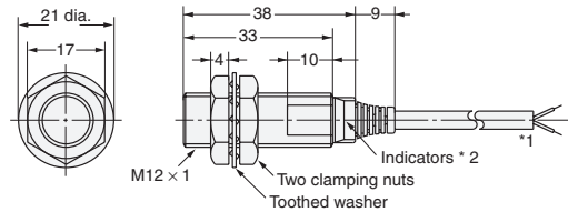
Diagram 5 E2E-X3D□ E2E-X2E□/F□
