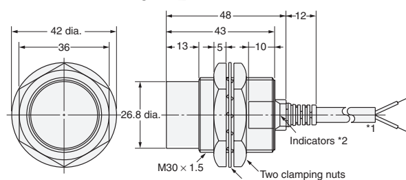
Diagram 13 E2E-X20MD□/E2E-X18ME□/F□ E2E-X18MY□
