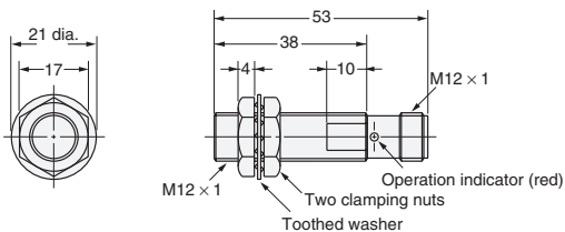
Diagram 18 E2E-X2Y□-M1
