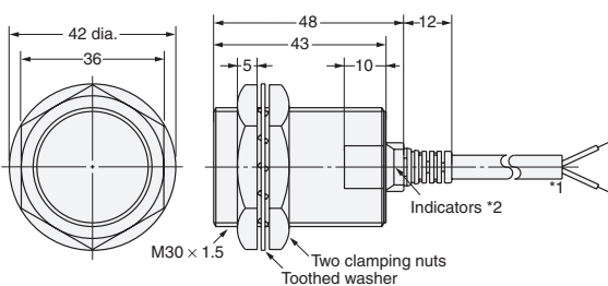
Diagram 12 E2E-X10D□/E2E-X10E□/F□ E2E-X10Y□/E2E-X10T1
