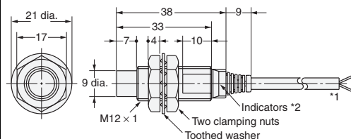
Diagram 6 E2E-X8MD□ E2E-X5ME□/F□
