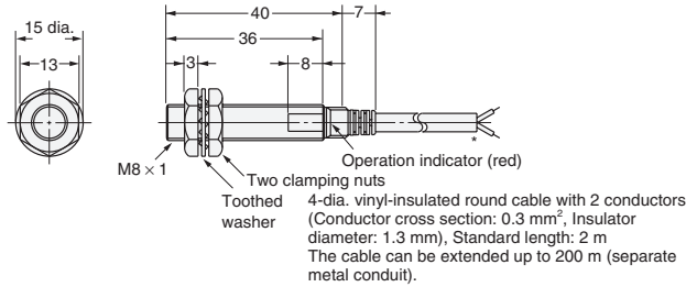
Diagram 5 E2E-X3D□ E2E-X2E□/F□
