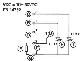
Wiring diagram 441
