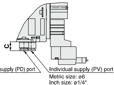
Individual SUP port dimensions (Option symbol: -L)*2
