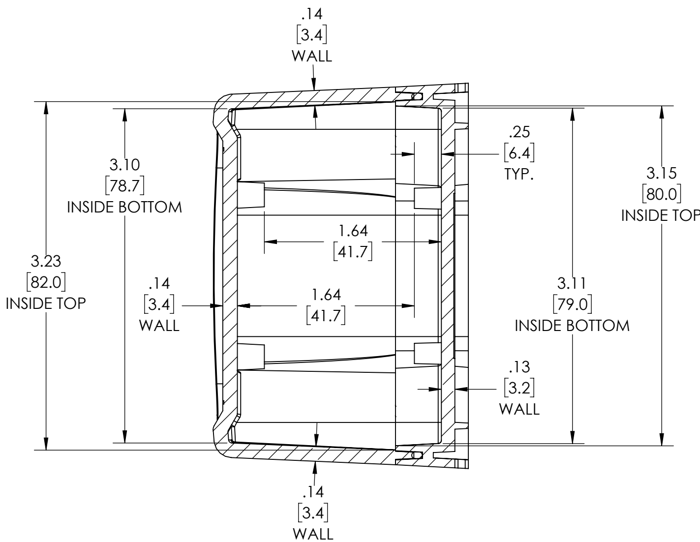
SECTION A-A SCALE 2 : 1.75
