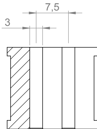
SCHNITT A-A
