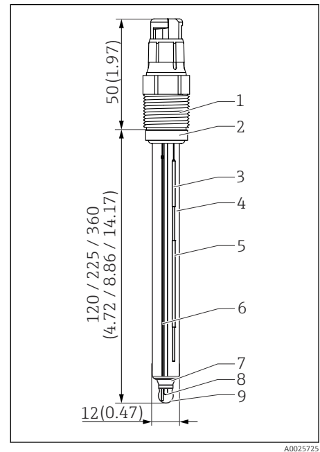
9 CPS11D-7BTxx, with ion trap
