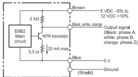
E6B2-CWZ3E
