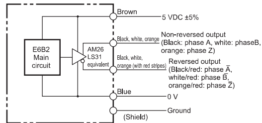
E6B2-CWZ1X
